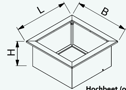
Hochbeet (ohne Boden)
