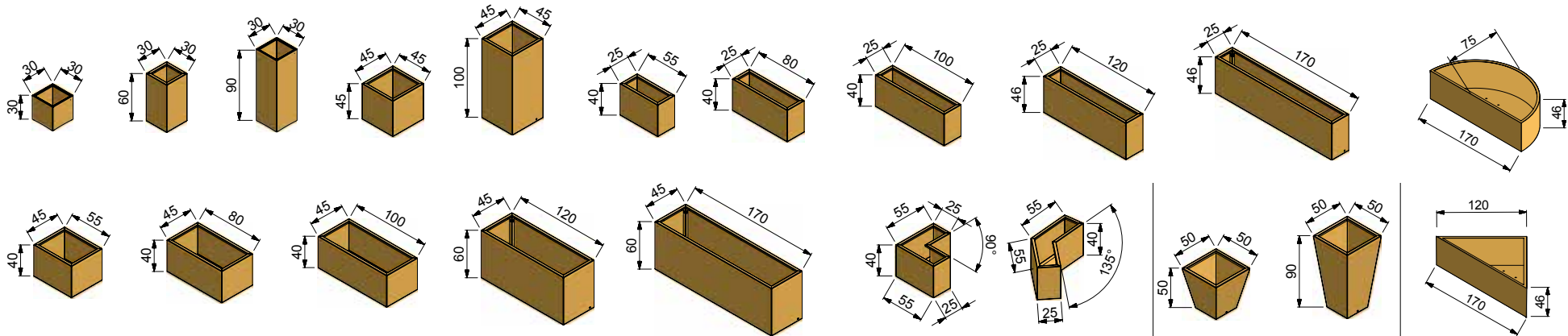
Pflanztrog Ergo klein
